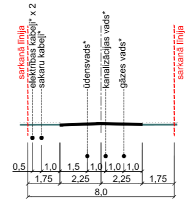
Projektētā ceļa šķersprofils M 1:200 (*ceļa profilā norādītie inženiertīkli ir plānotie perspektīvie tīkli, kas ir obligāti realizējami pēc pilsētas centralizēto tīklu izbūves)
